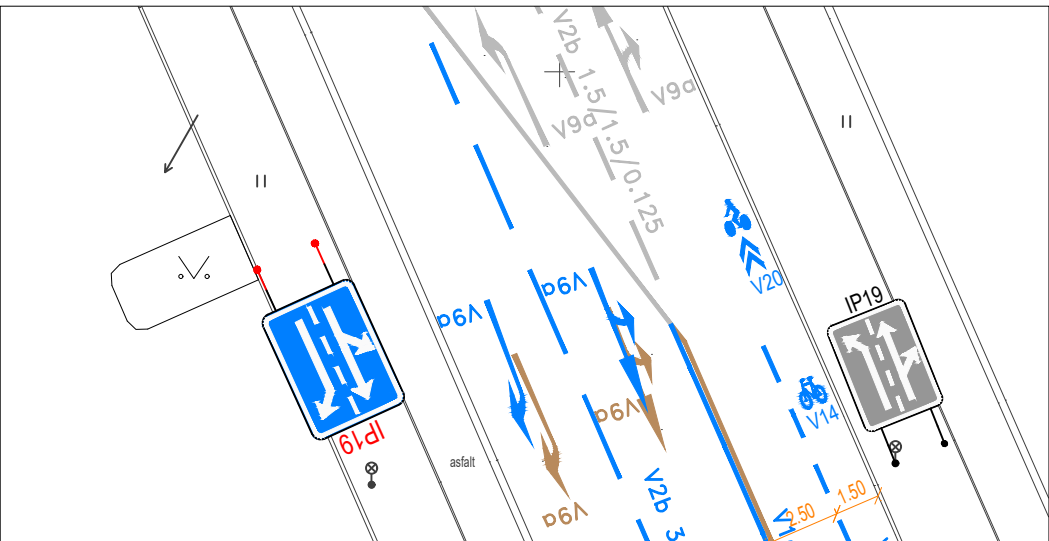
VÝŘEZ 1: Poloha nového vodorovného dopravního značení ve vzdálenosti cca 45 m před stopčarou SS VA
