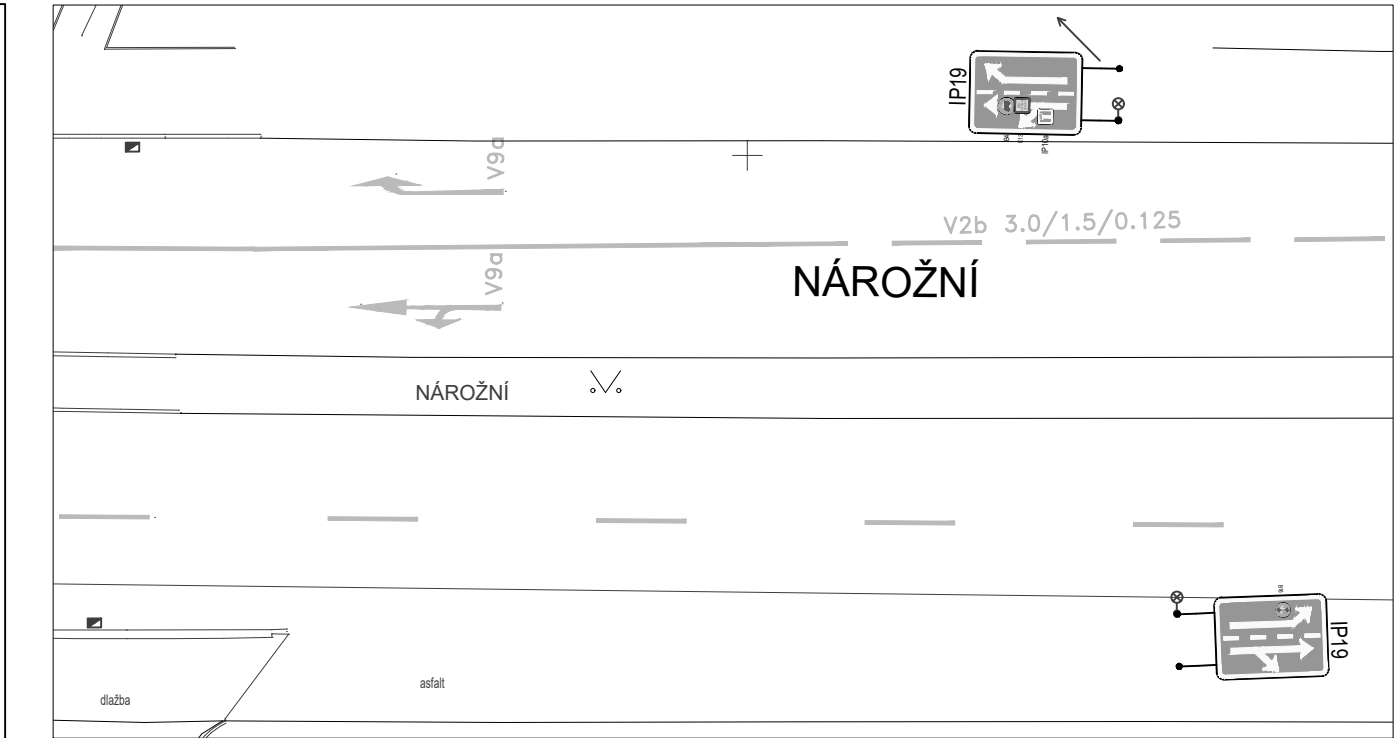
VÝŘEZ 2: Poloha stávajících svislého dopravního značení ve vzdálenosti cca 100 m před stopčarou SS VD
